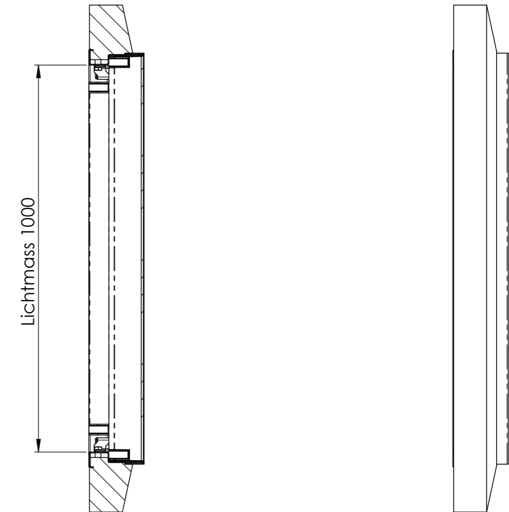
SCHNITT B-B
